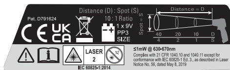
Etiqueta de advertencia en la parte lateral del termómetro
